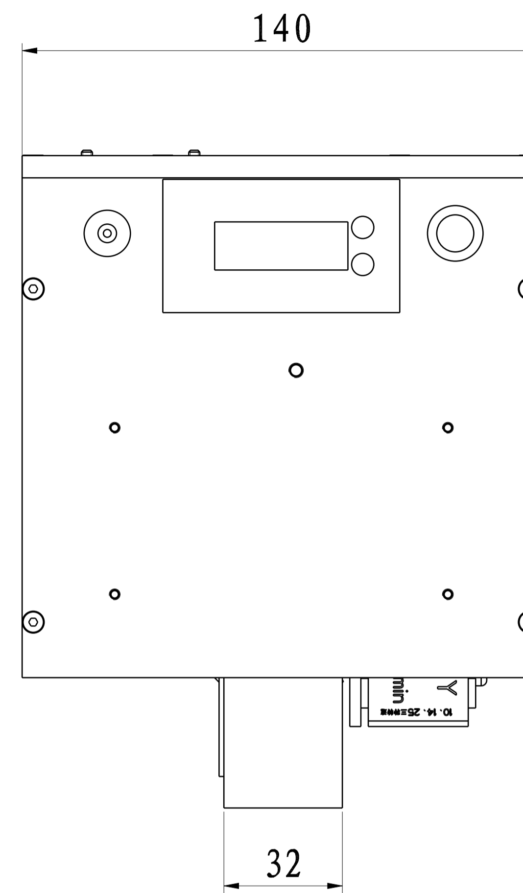
左视图
