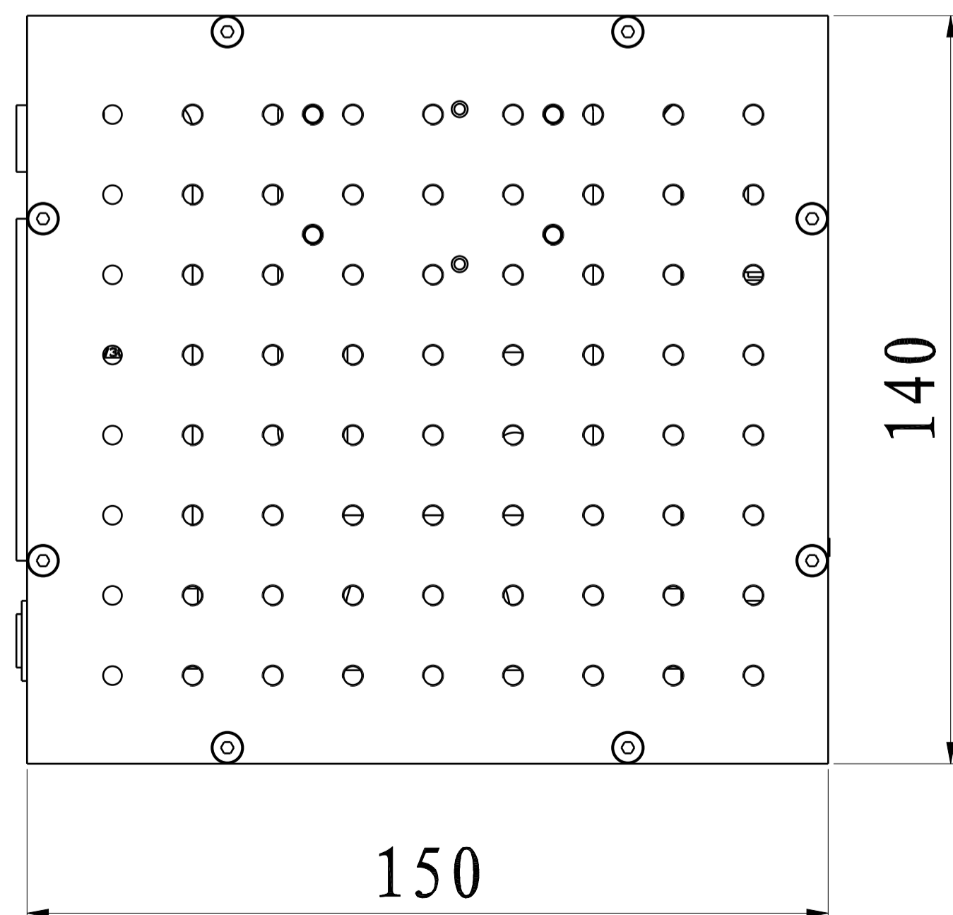
俯视图
