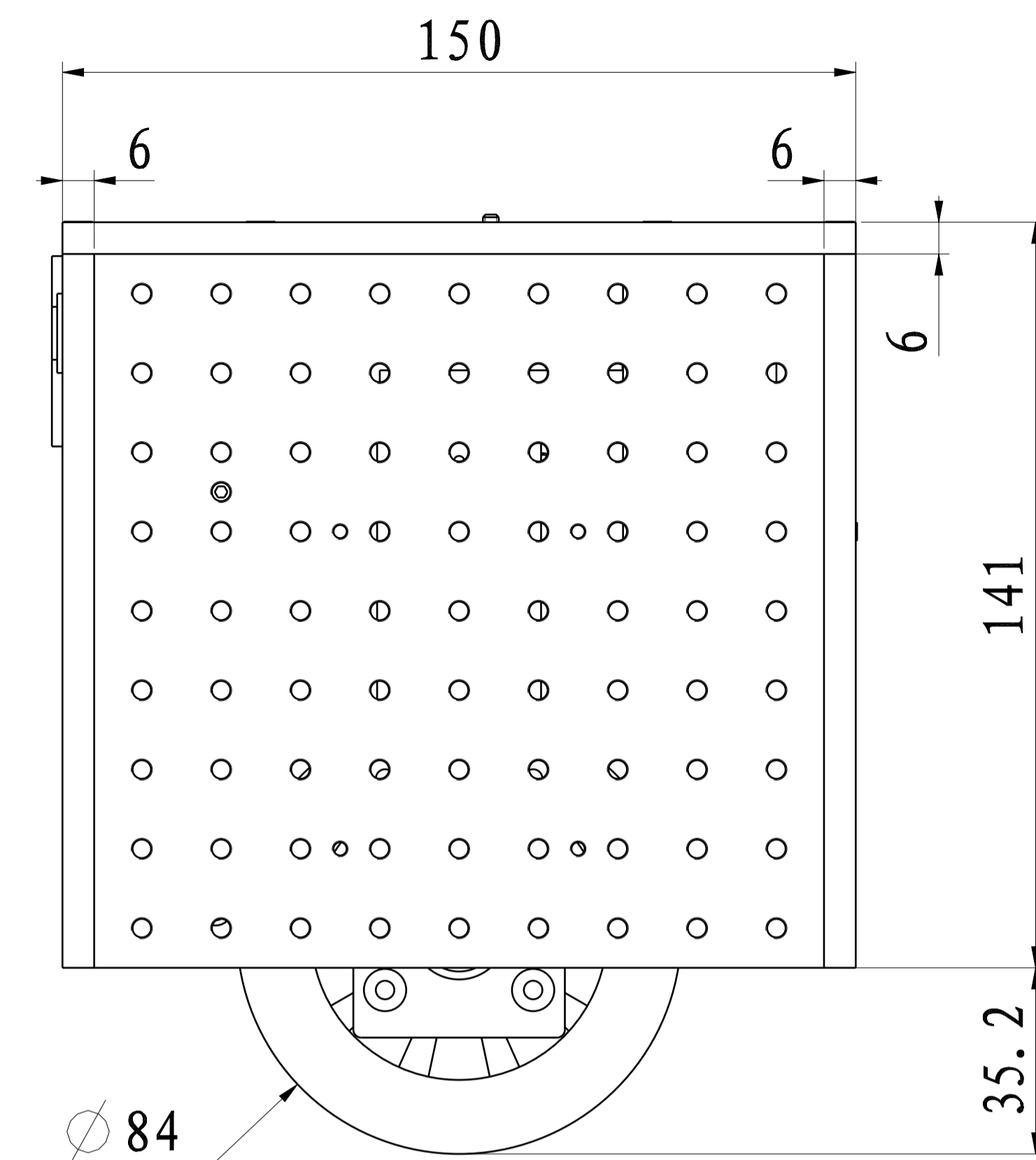
主视图
